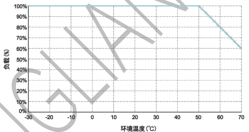
负载VS环境温度
